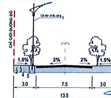
MẶT CẮT 1-1
