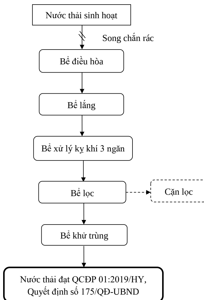
Hình 3.2. Sơ đồ hệ thống xử lý nước thải sinh hoạt
