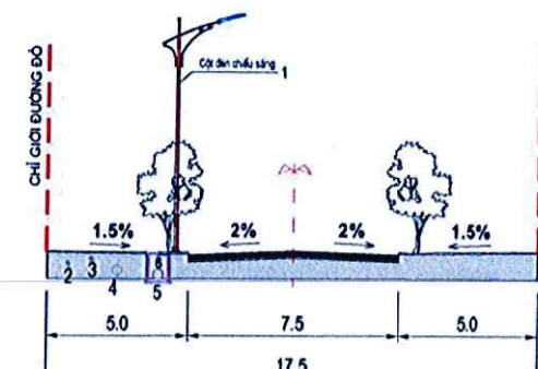
MẶT CẮT 3-3
