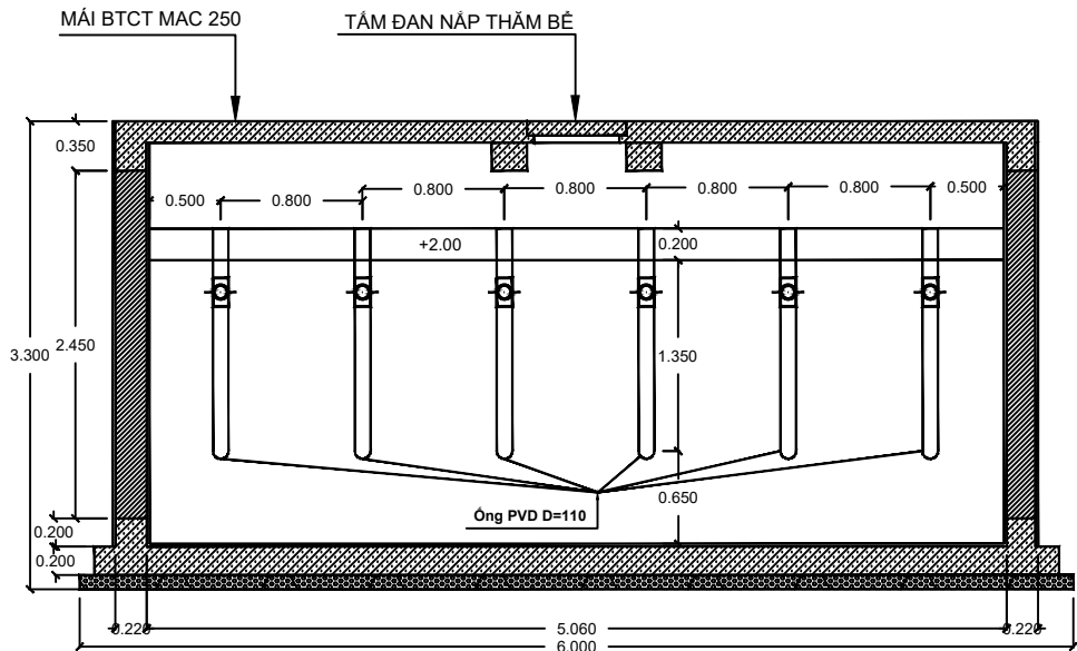
CẮT NGANG BỂ LẮNG (CẮT 1-1)
