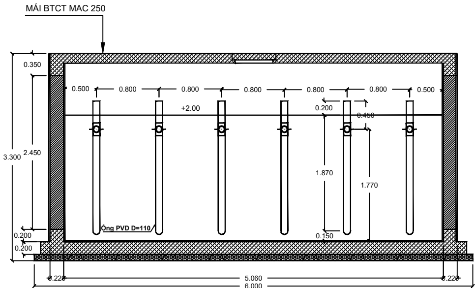
CẮT NGANG ABR (CẮT 2-2)
