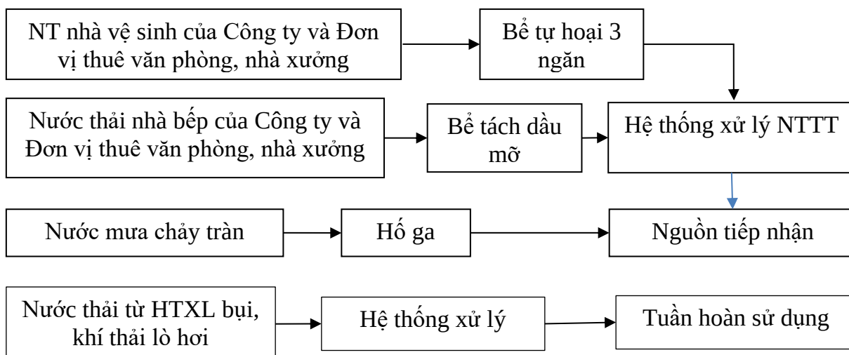
Hình 3.8. Sơ đồ phân luồng dòng thải của dự án
