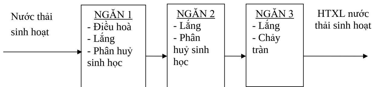
Hình 3.9. Công nghệ xử lý nước thải sinh hoạt bằng bể tự hoại 3 ngăn
