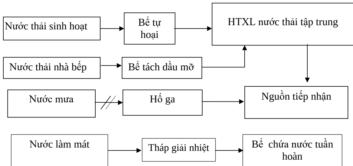
Hình 3.3. Sơ đồ phân luồng dòng thải của dự án
