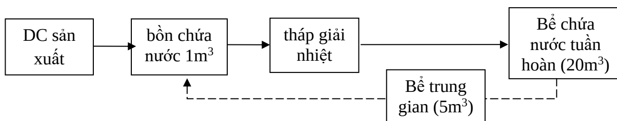
Hình 3.5. Sơ đồ hệ thống tuần hoàn nước làm mát của nhà máy
