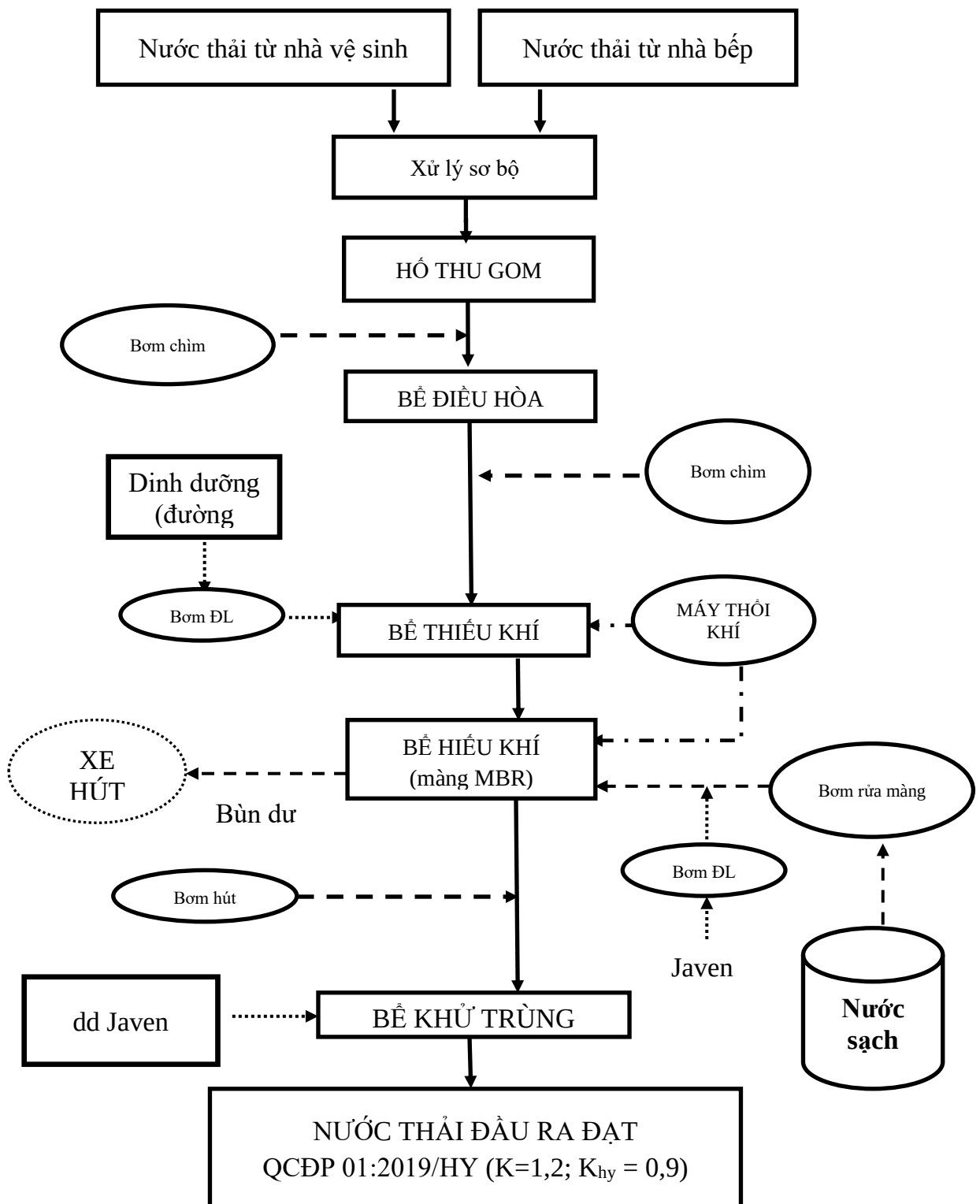
Hình 3.6. Sơ đồ công nghệ xử lý nước thải của Công ty
