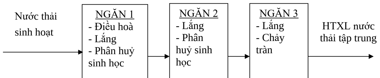
Hình 3.4. Công nghệ xử lý nước thải sinh hoạt bằng bể tự hoại 3 ngăn
