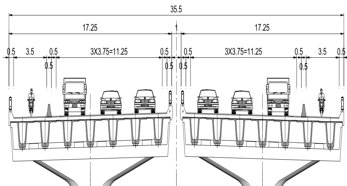
Mặt cắt ngang cầu dẫn
