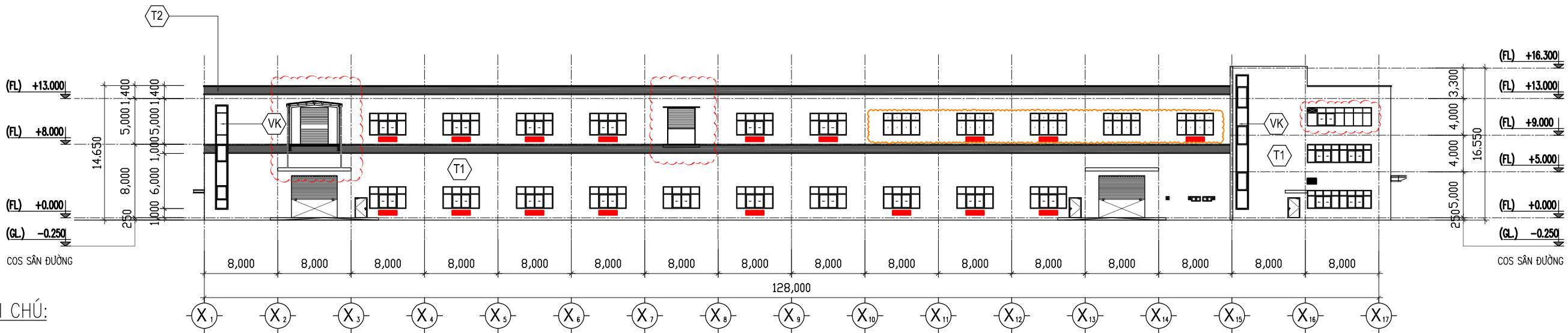
MẶT ĐỨNG TRỰC X1-X17/ X1-X17轴立面
