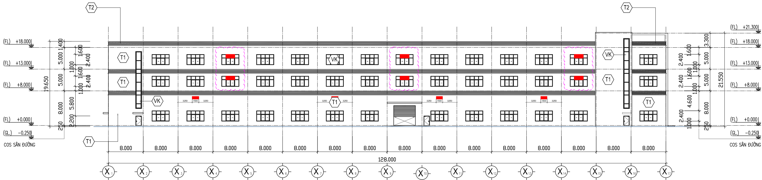
MẶT ĐỨNG TRỰC X1-X17/ X1-X17轴立面
