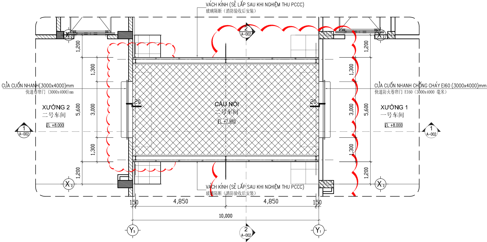
MẶT BẰNG CẦU NỐI/ 连桥平面图 1/75
