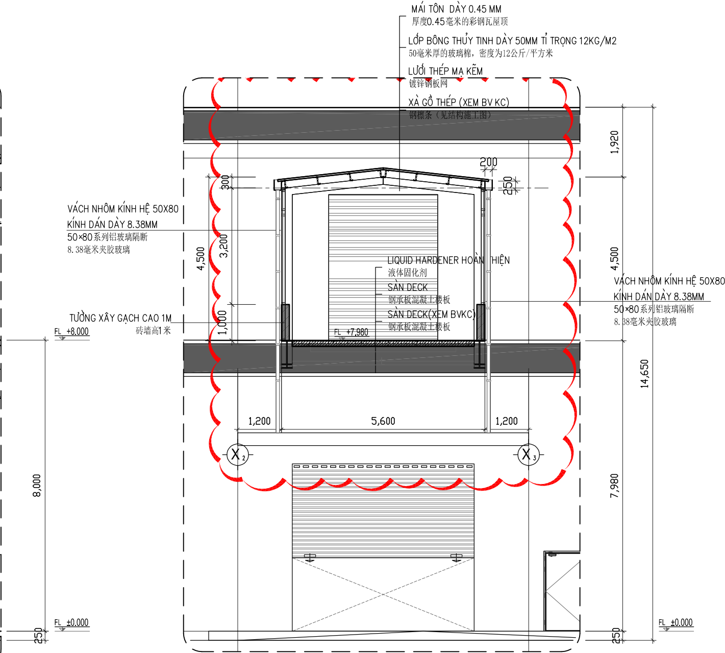
MẶT CẮT 2-2/ 2-2 剖面图 1/75
