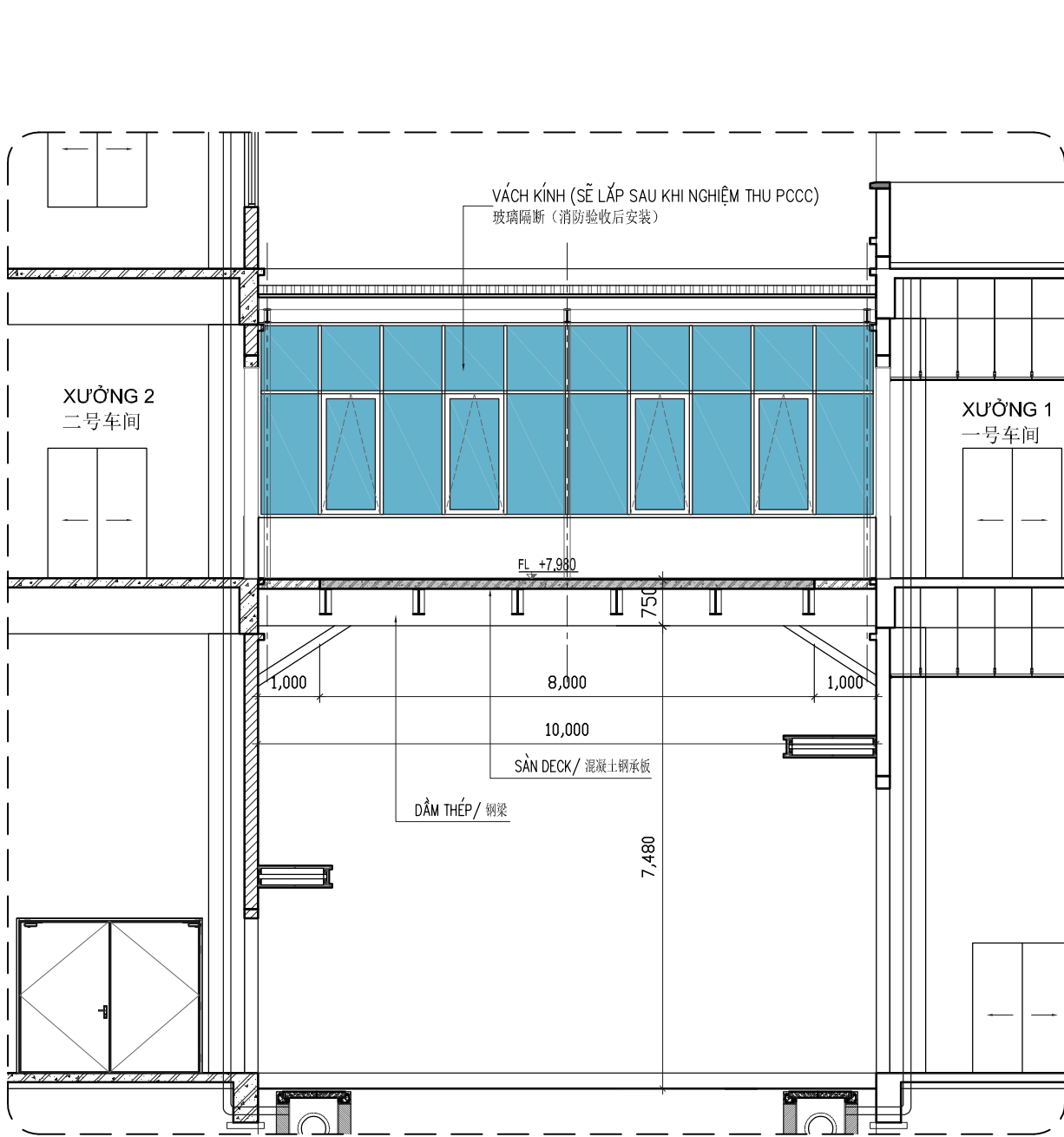
MẶT CẮT 1-1/ 1-1 剖面图 1/75
