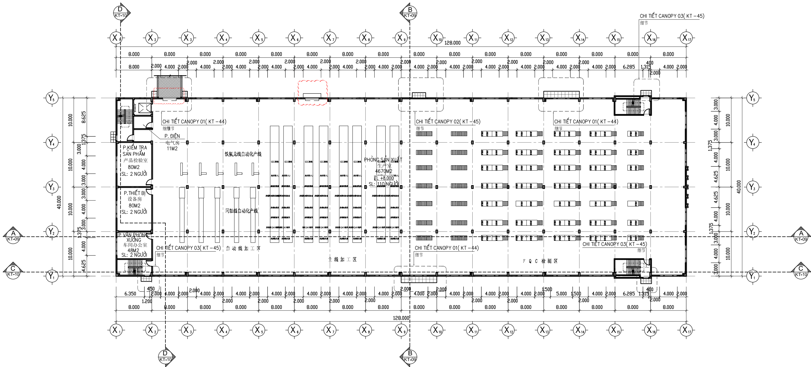
MẶT BẰNG TẦNG 2 / 2层平面
