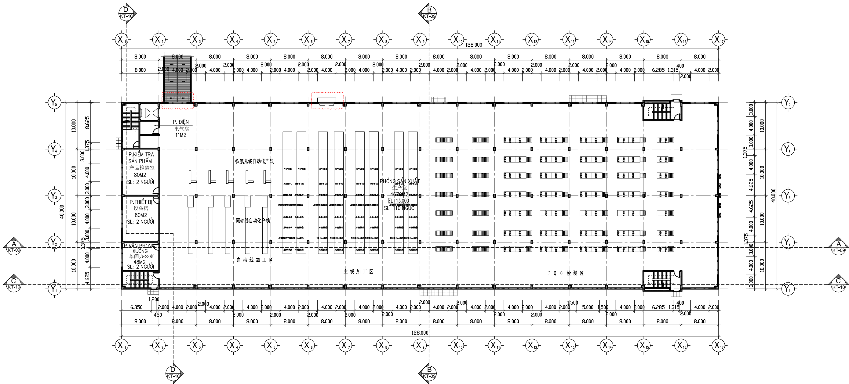
MẶT BẰNG TẦNG 3 / 3层平面
