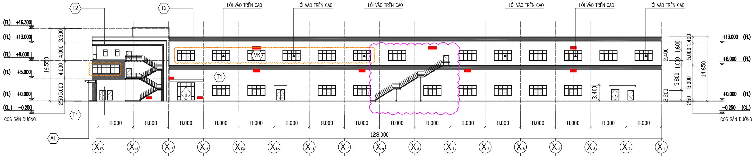
MẶT ĐỨNG TRỰC X17-X1/ X17-X1轴立面
