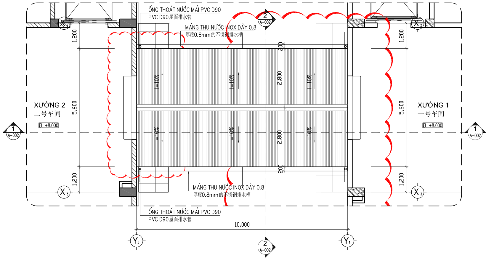
MẶT BẰNG MÁI CẦU NỐI/ 连桥屋顶平面图 1/75
