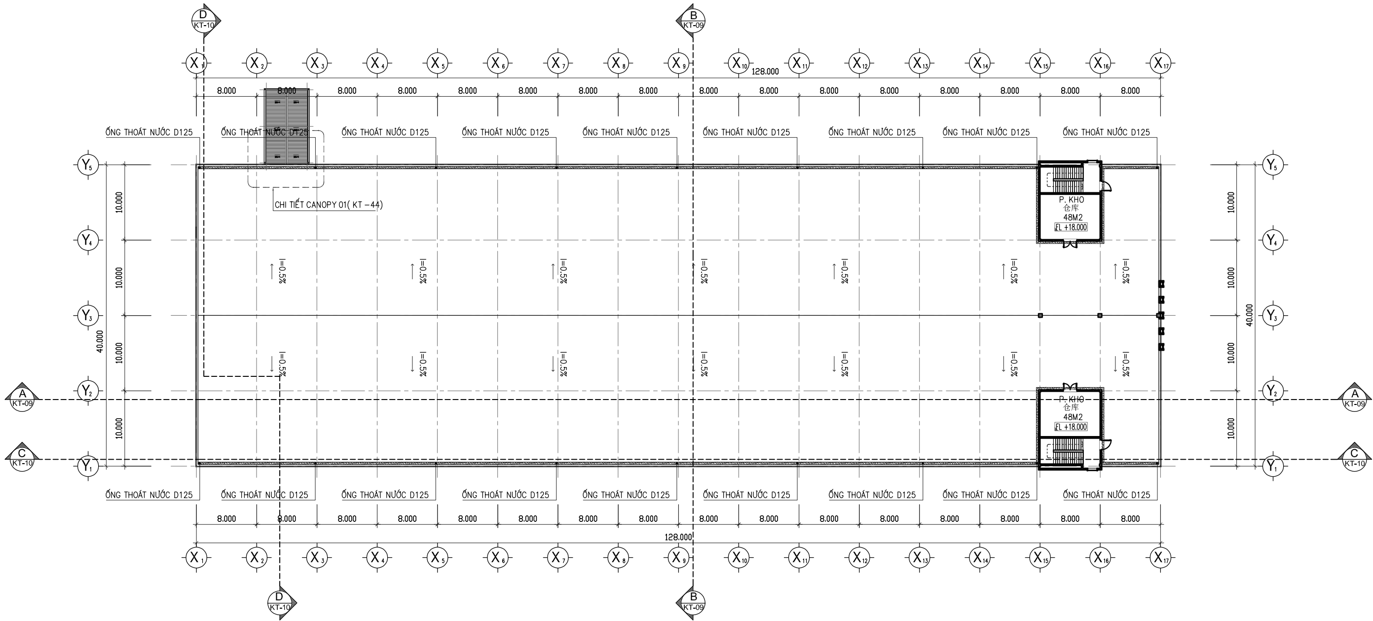
MẶT BẰNG TẦNG TUM / 楼梯间平面
