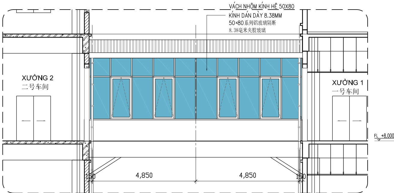
MẶT ĐỨNG TRỤC Y5-Y1/ Y5-Y1轴立面图 1/75
